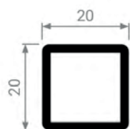
Профіль квадратний
